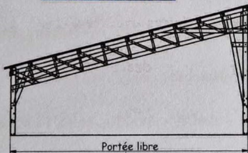
APPENTIS SEULS
